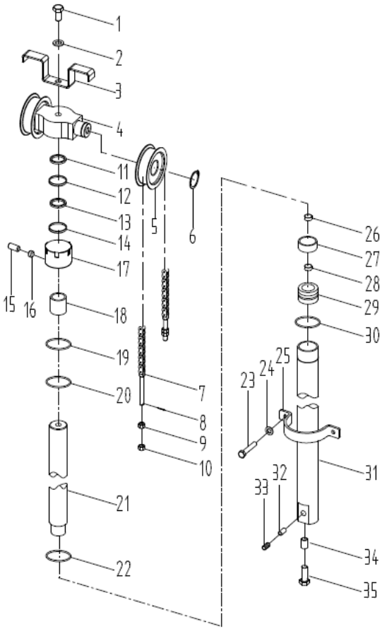
图105/FIG105. 前起升油缸(二级全自由)/FRONT LIFT CYLINDER(FULL FREE 2-STAGE MAST)
