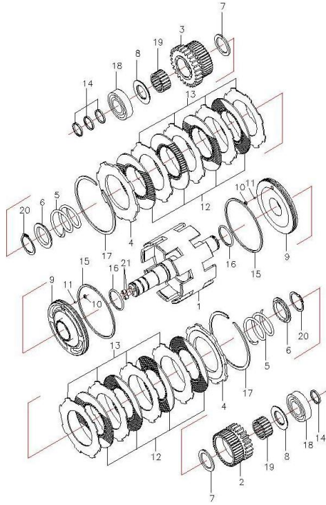
图7 液力离合器
